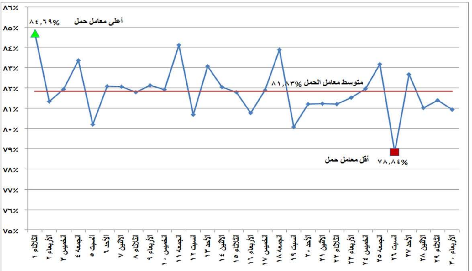
شكل (١٢) إجمالي معامل الحمل لوحدات الانتاج خلال شهر نوفمبر ٢٠١٦
