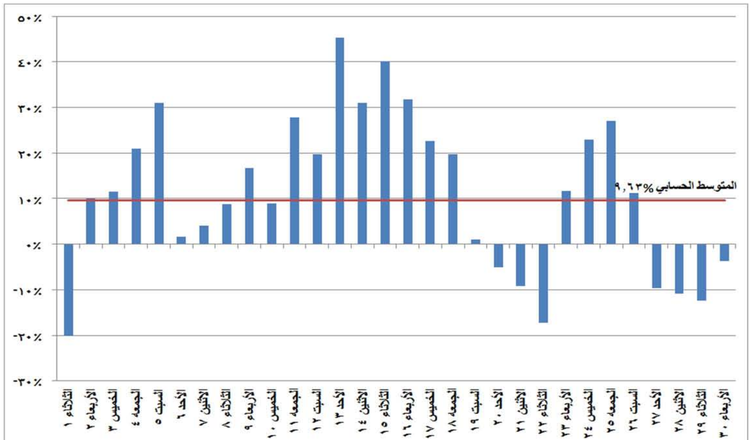
شكل (٢٢) نسب التغير في استخدام المصادر غير الحرارية في إنتاج الطاقة الكهربائية خلال شهر نوفمبر ٢٠١٦ مقارنة بالشهر المماثل من العام السابق
