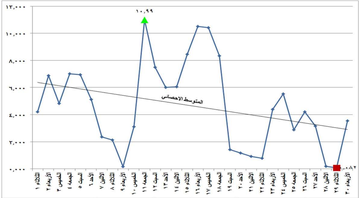
شكل (٢٥) الطاقة الكهربائية المنتجة من الرياح والشمس خلال شهر نوفمبر ٢٠١٦
