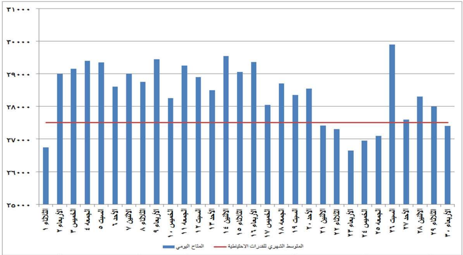
شكل (٢٧) القدرات المتاحة يوميا والمتوسط الشهري للقدرات الاحتياطية خلال شهر نوفمبر ٢٠١٦
