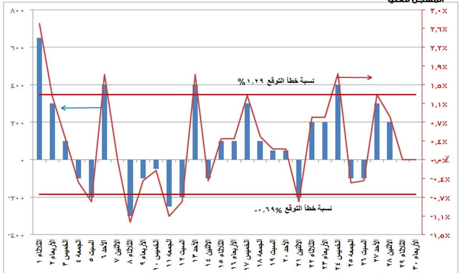
شكل (١٠) الفرق بين الحمل الأقصى المتوقع والمسجل فعليا ونسبة الفرق إلى الحمل المسجل فعليا خلال شهر نوفمبر ٢٠١٦
