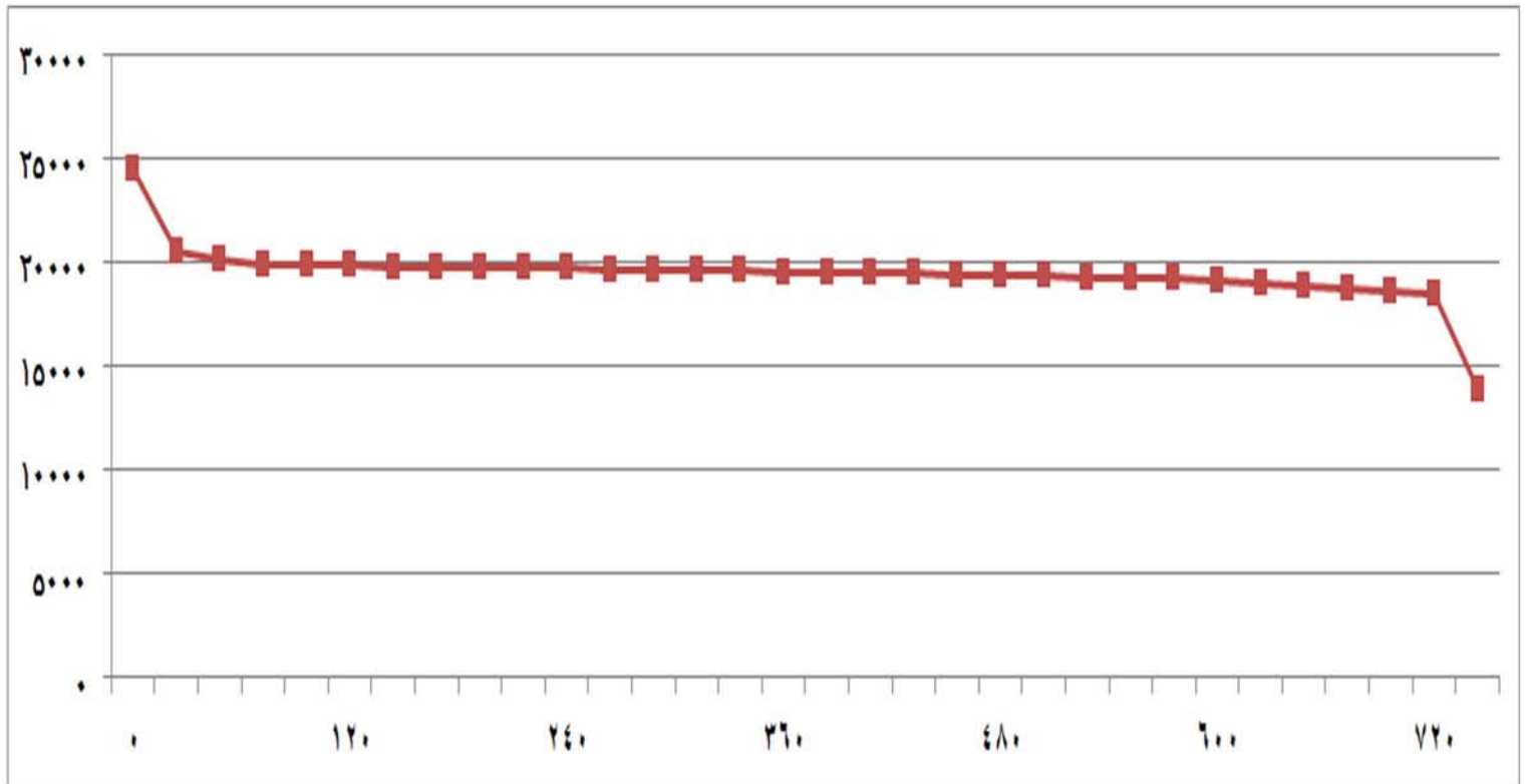
شكل (٨) المنحنى الشهري لفترة الحمل نوفمبر ٢٠١٦
