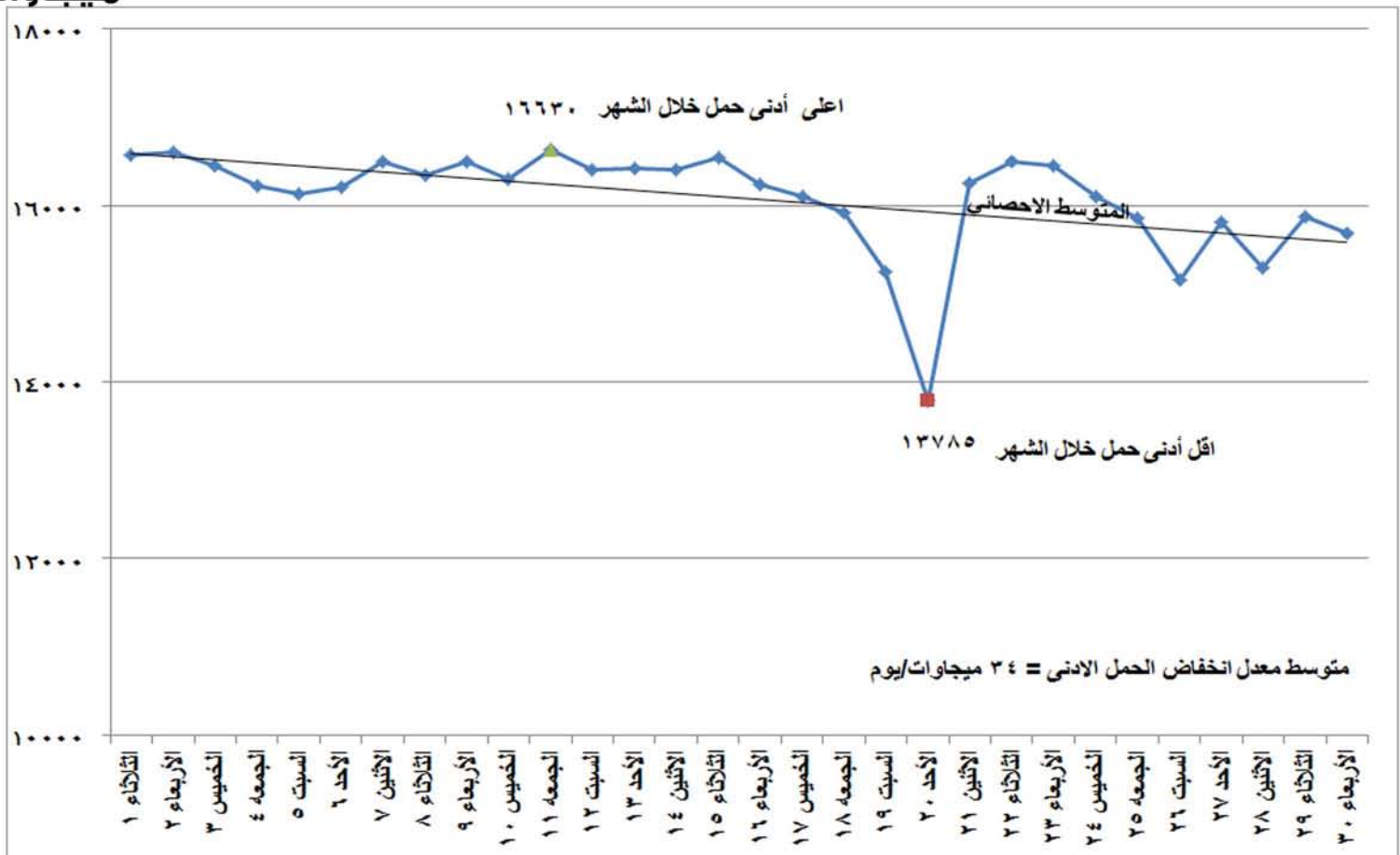
شكل (٢) تطور الحمل الادنى اليومي خلال شهر نوفمبر ٢٠١٦
