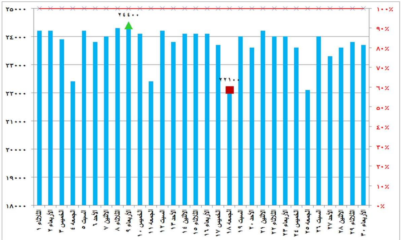
شكل (٥) قدرات الانتاج المتاحة ونسبتها للحمل الأقصى خلال شهر نوفمبر ٢٠١٦
