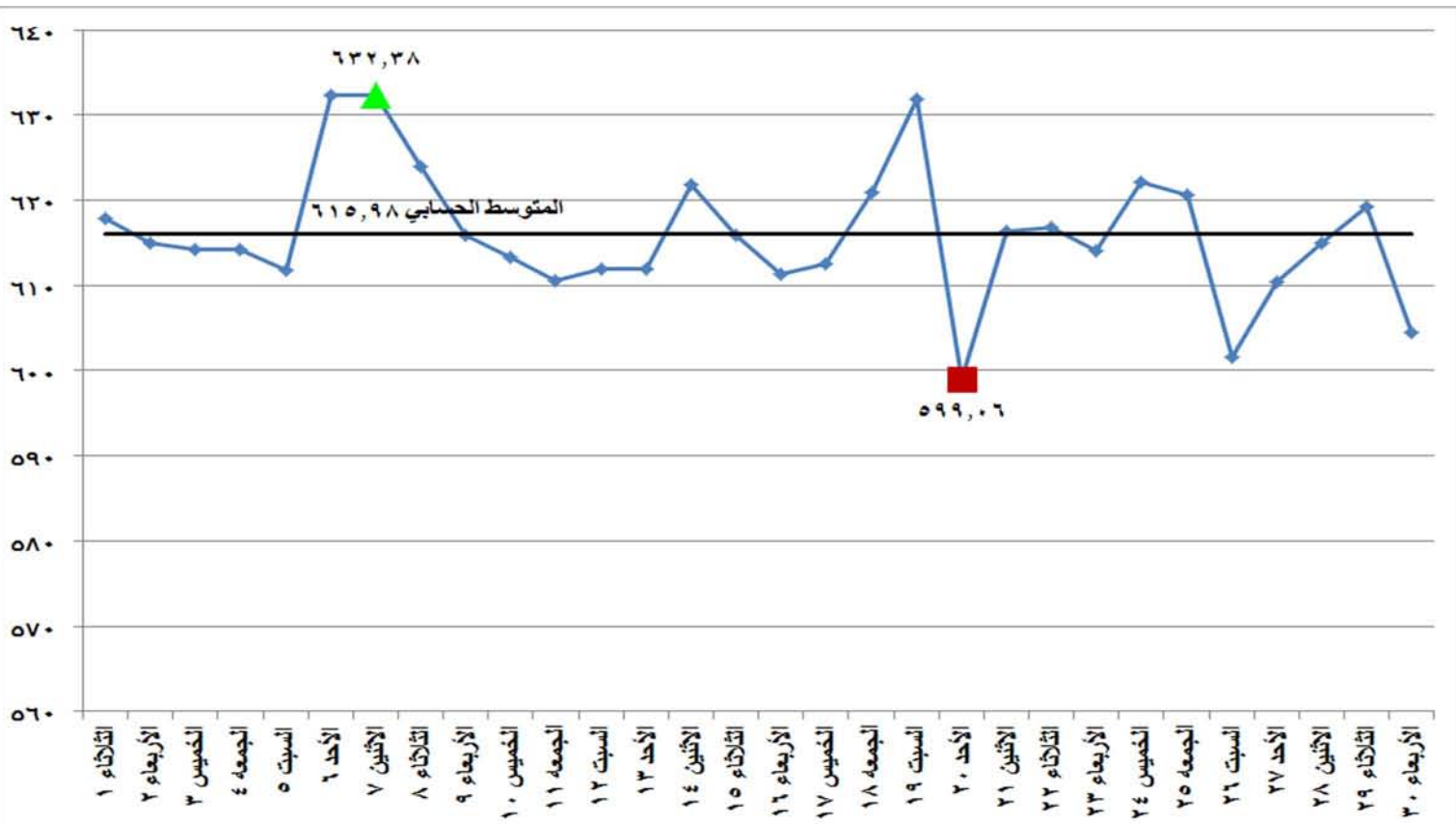
شكل (١٤) معامل انبعاثات غاز ثاني اكسيد الكربون المكافئ على مدى شهر نوفمبر ٢٠١٦
