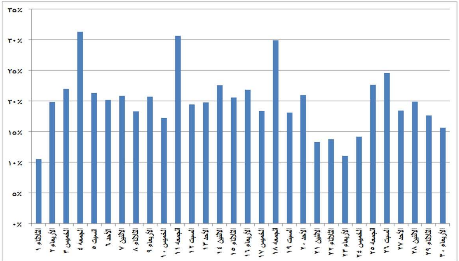
شكل (٢٨) نسب الفائض للحمل الاقصى المسجل يوميا خلال شهر نوفمبر ٢٠١٦
