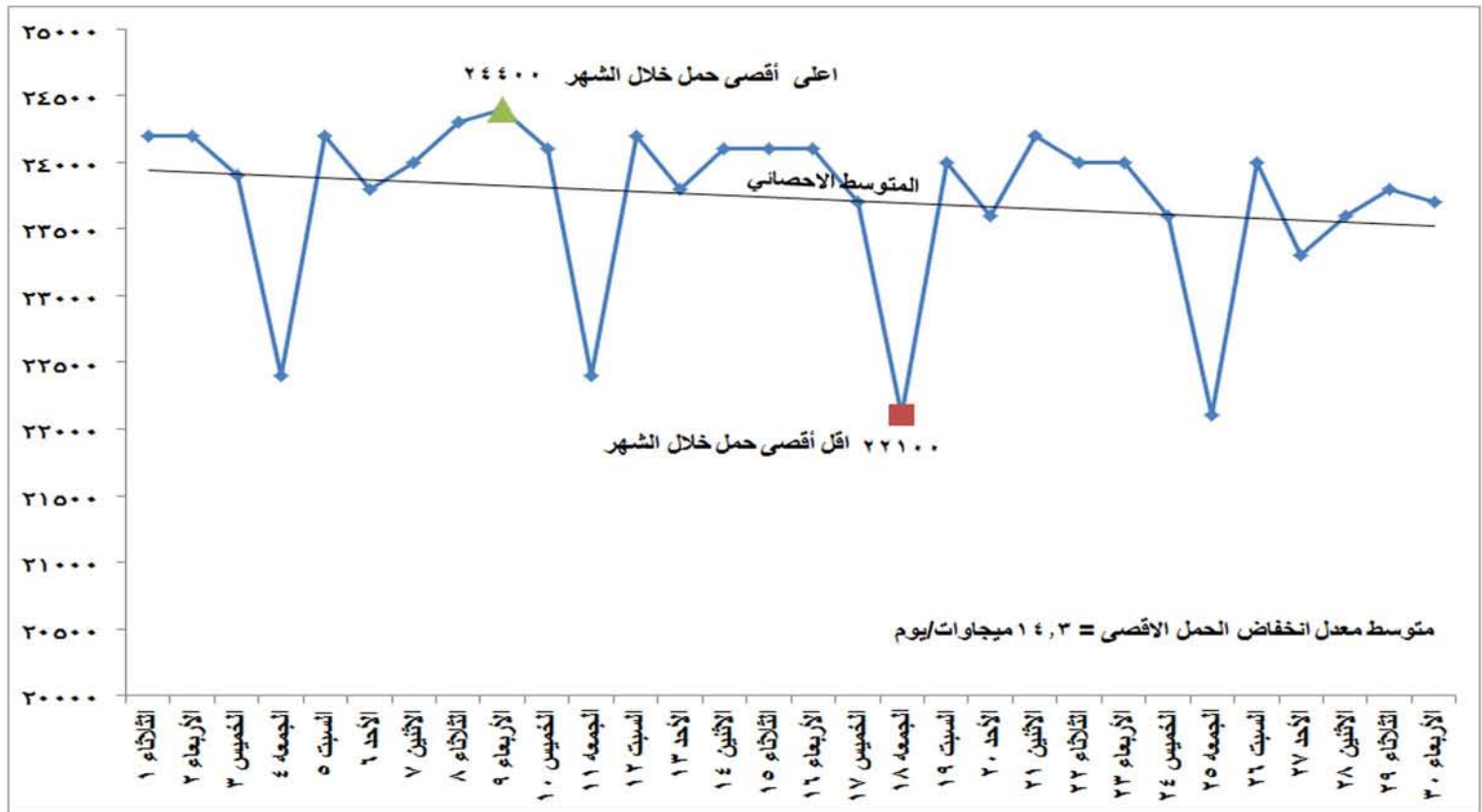
شكل (١) تطور الحمل الاقصى اليومي خلال شهر نوفمبر ٢٠١٦
