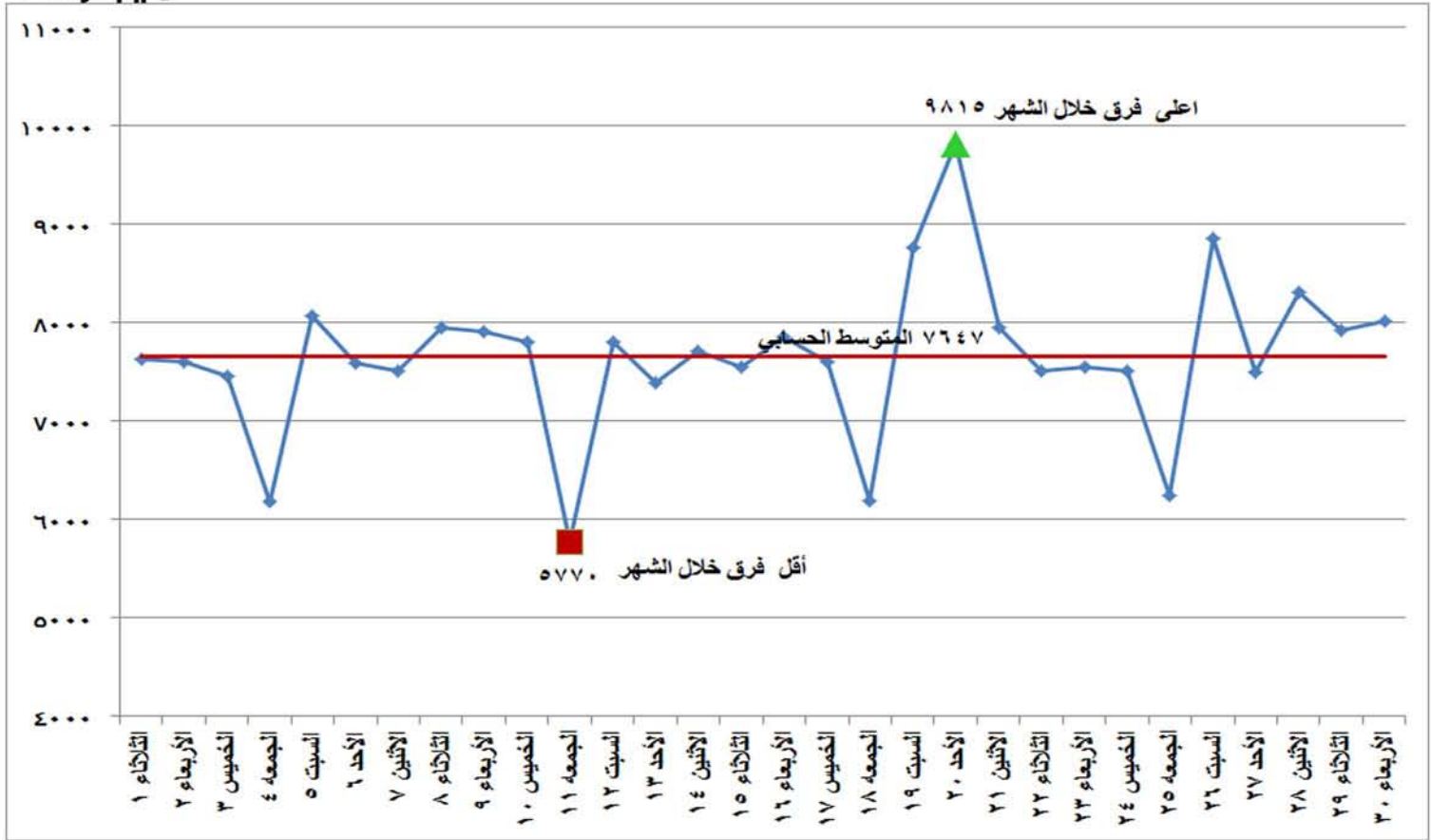
شكل (٣) الفرق بين أقصى وأدنى حمل خلال شهر نوفمبر ٢٠١٦
