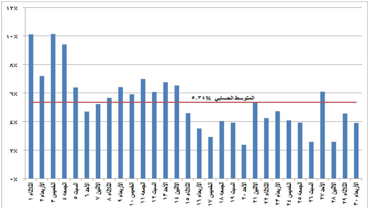
شكل (١٦) نسب التغير في الطاقة الكهربائية المنتجة خلال شهر نوفمبر ٢٠١٦ مقارنة بالشهر المماثل من العام السابق
