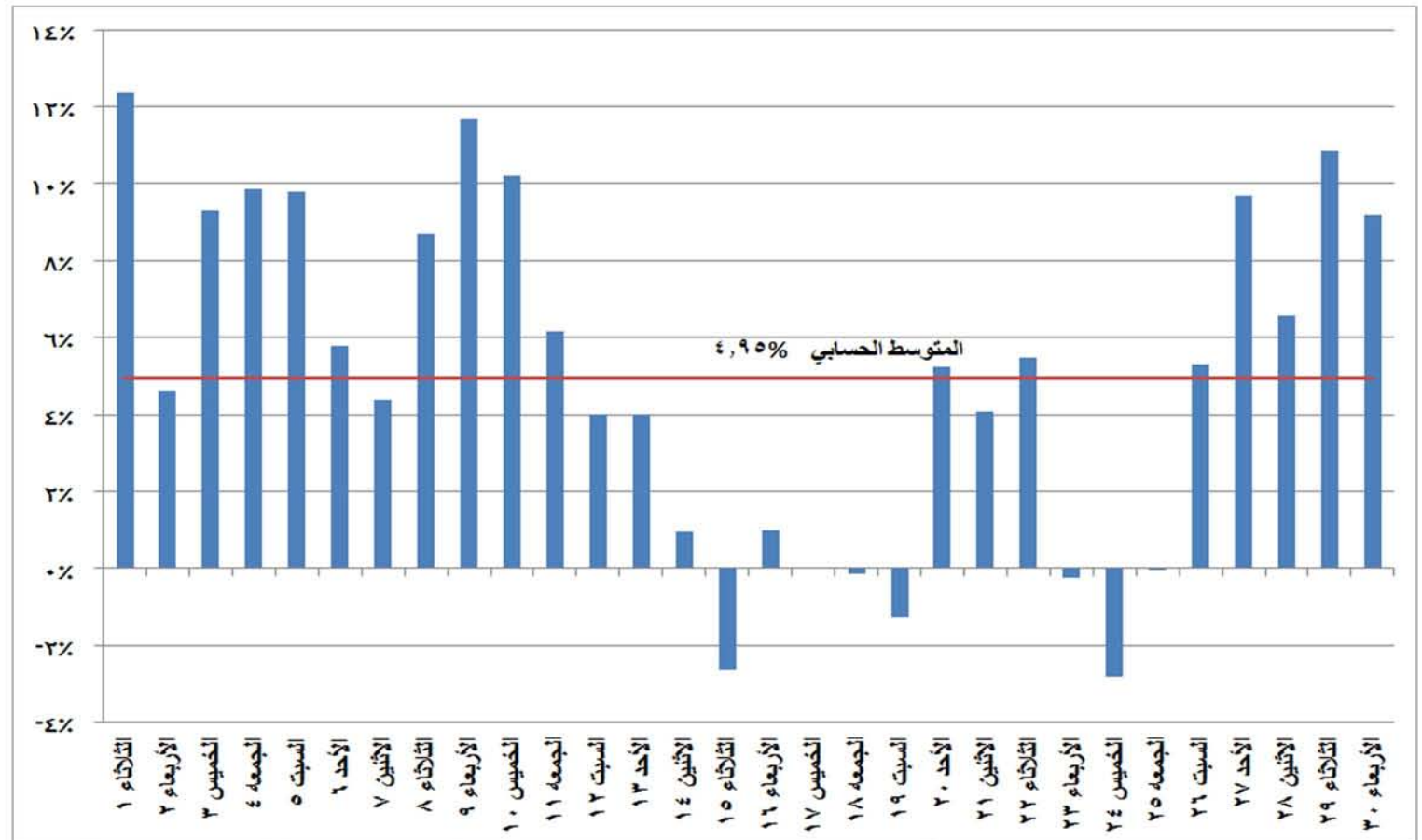
شكل (١٨) نسب التغير في استخدام الغاز الطبيعي في إنتاج الطاقة الكهربائية خلال شهر نوفمبر ٢٠١٦ مقارنة بالشهر المماثل من العام السابق
