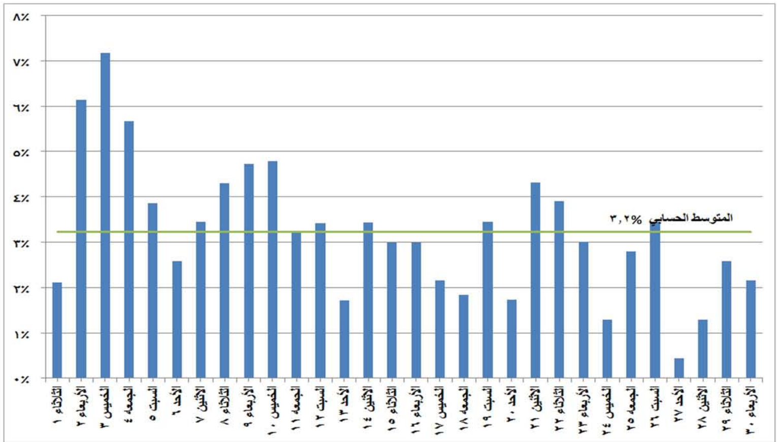
شكل (٩) النسب المئوية للتغير في الحمل الاقصى خلال شهر نوفمبر ٢٠١٦ مقارنة باليوم المماثل من العام الماضي
